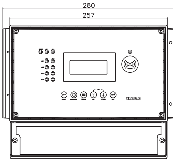
정면도
