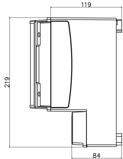
측면도
