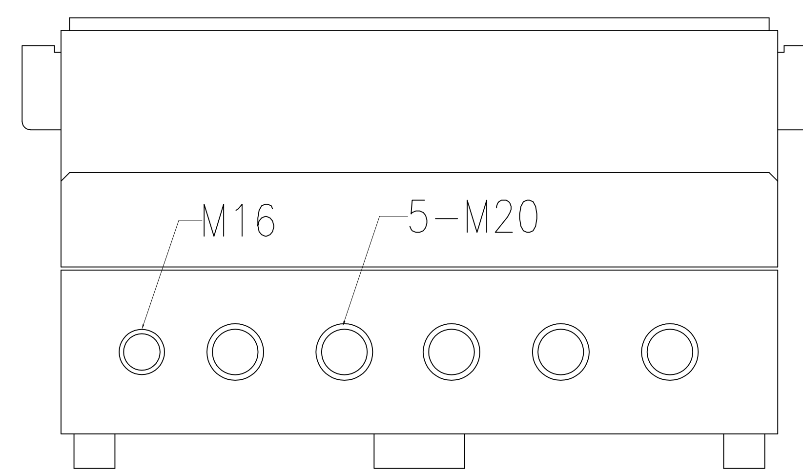
( 정면도 )
